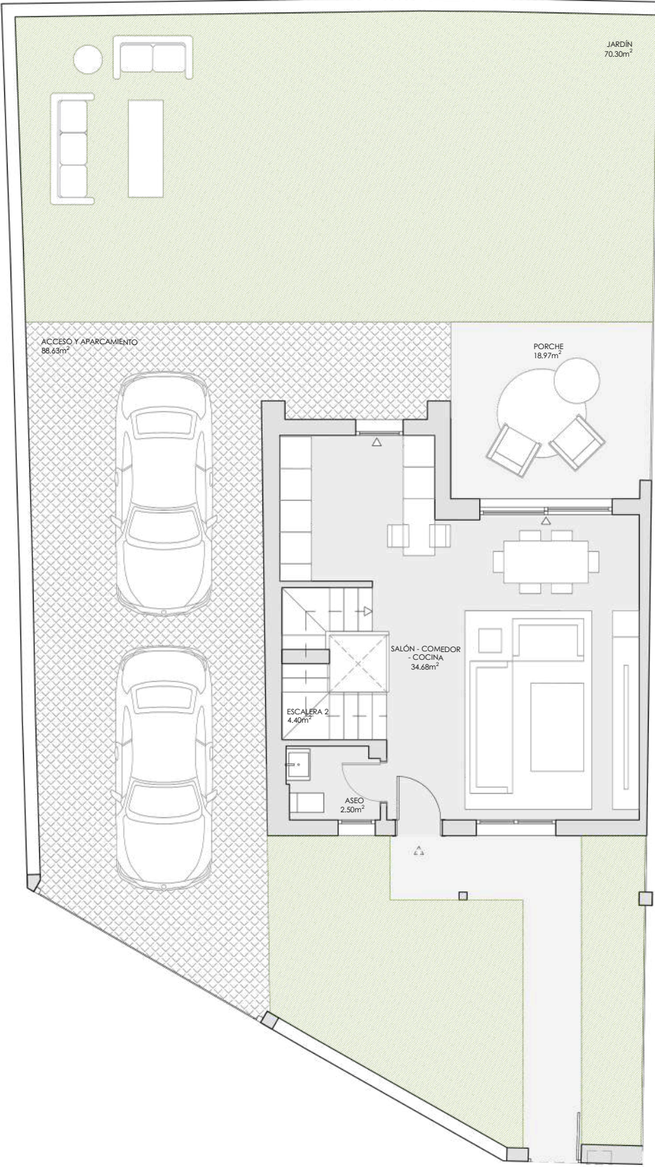
PLANTA BAJA
