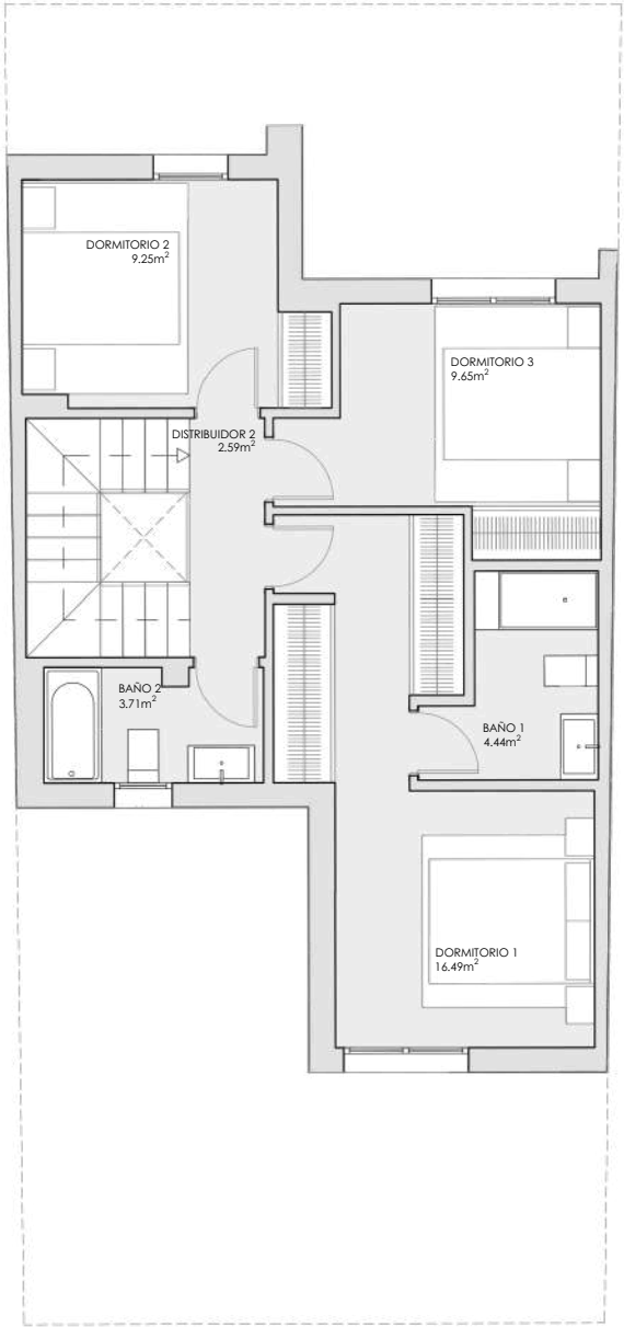
PLANTA PRIMERA
