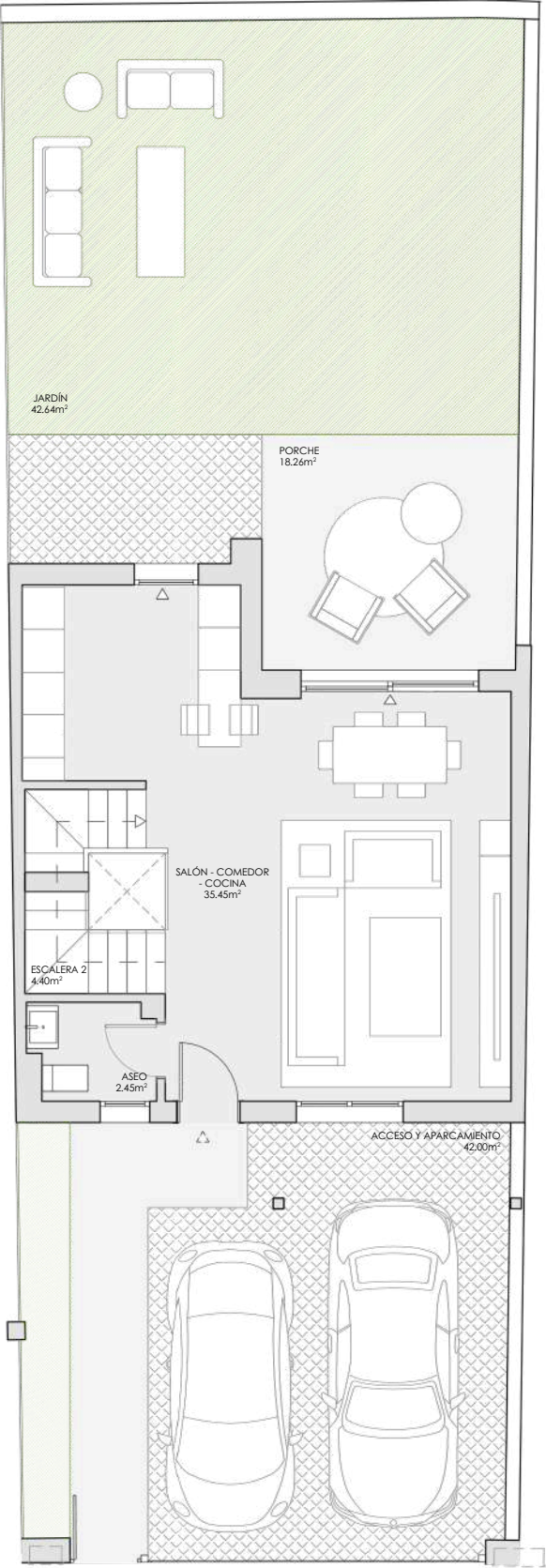
PLANTA BAJA
